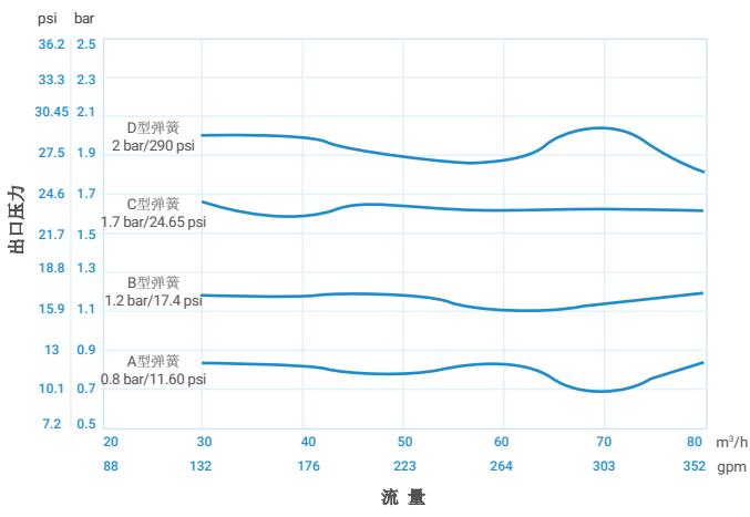
→ 出口压力 - 流量 曲线
