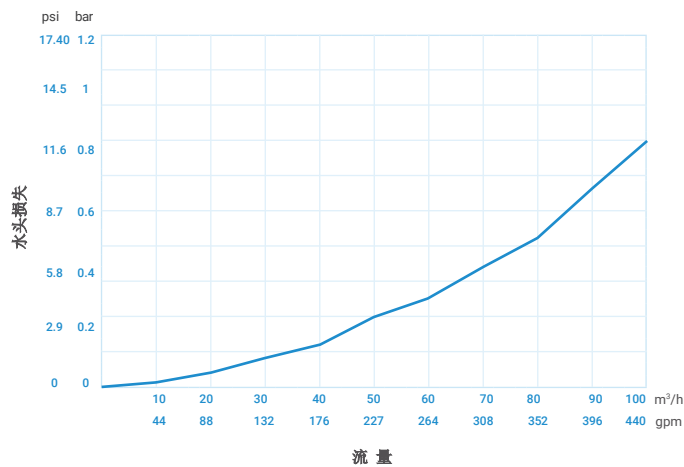
→ 水头损失 - 流量 曲线
