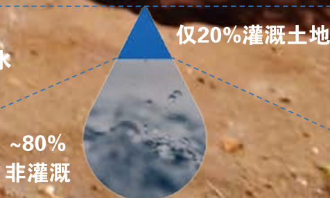
灌溉面积占耕地的百分比
