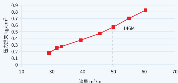
冲洗压力损失曲线图
