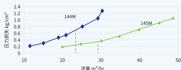
冲洗压力损失曲线图
